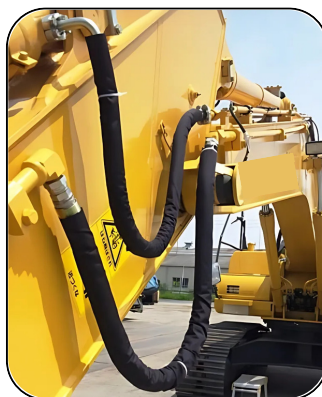
(Phần Ống thủy lực xi lanh gầu PC200)
